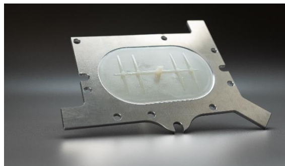
Abb. 1: Demonstrator eines Metall-Kunststoff-Verbundes
